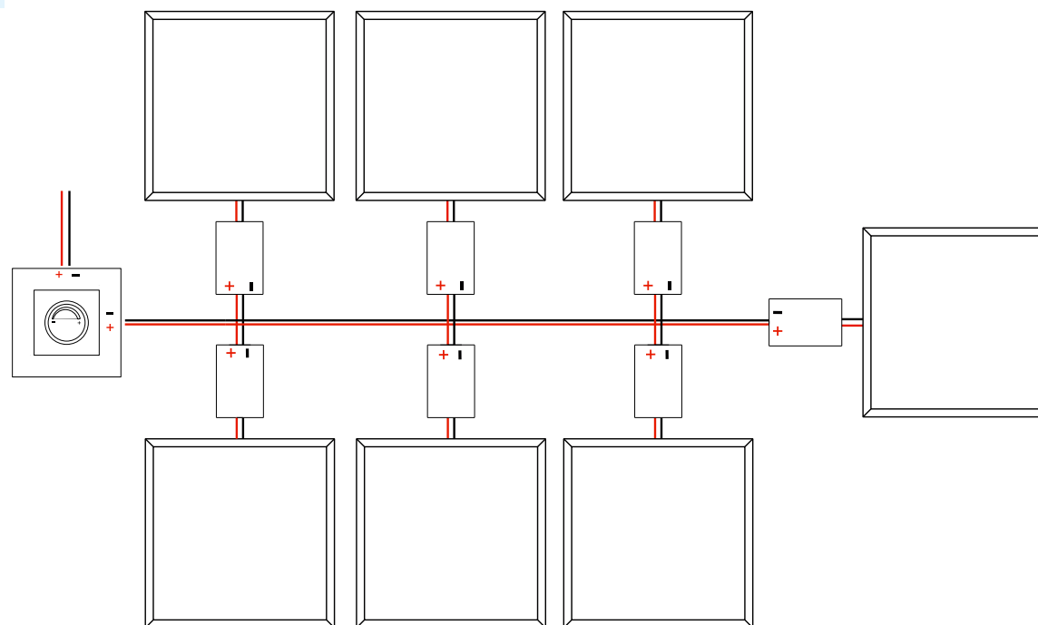
Схема подключения светильников к диммеру.
