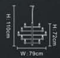
MT1710/30P SATIN NICKEL E14, 30xMAX. 7W(Energy-Saving) G9, 30xMAX. 40W
