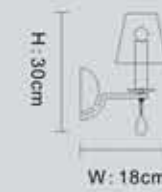
MT2176/1W CHROME E14,1 x Max.40W
