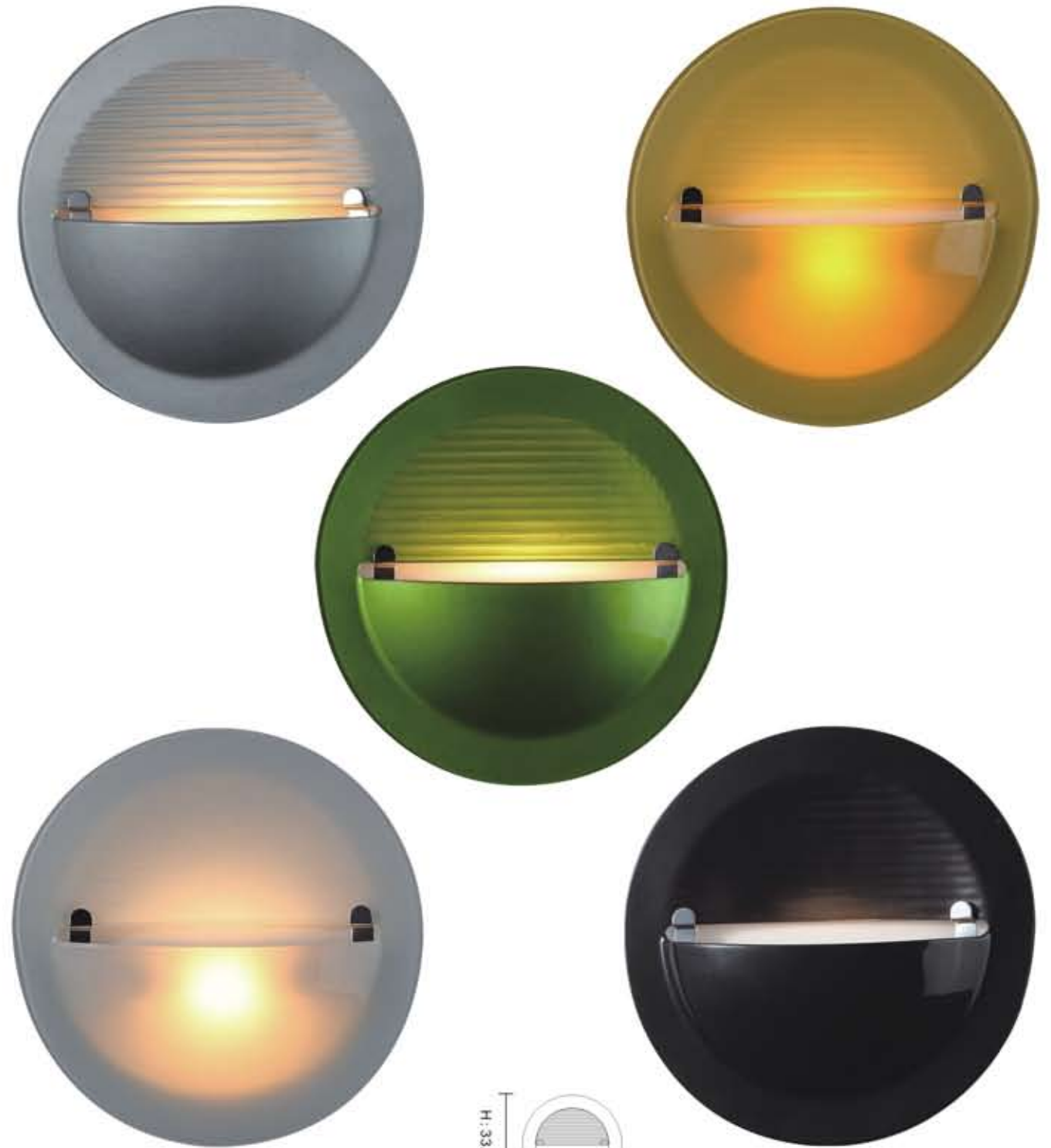
H: 33.5cm W: 33.5cm MT2323/1W WHITE & CHROME R7s,1 x Max.100W
