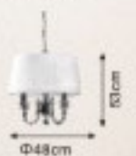
P9983/03B(PIG) E14 3x60W
