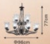
H6016/12A (ARS) E27 12x60W
