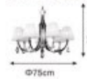
H8036/07B (CR) E14 7x60W
