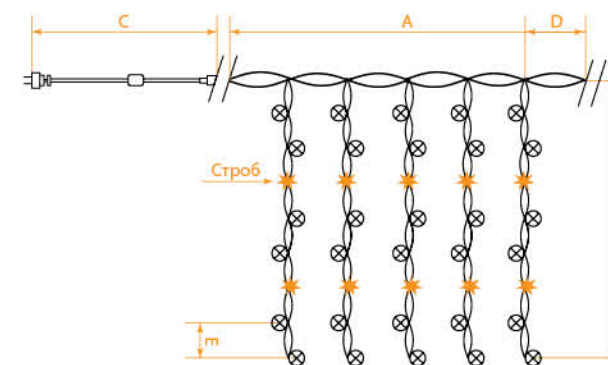
Схема
