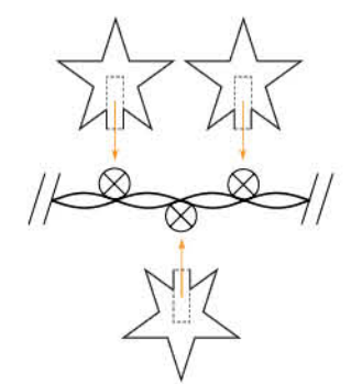
Схема крепления украшений на гирлянде
